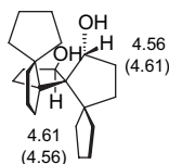
28 cis-cis
